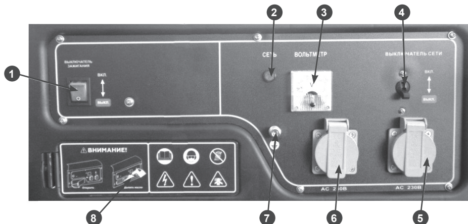
Рис. 3 Панель управления
